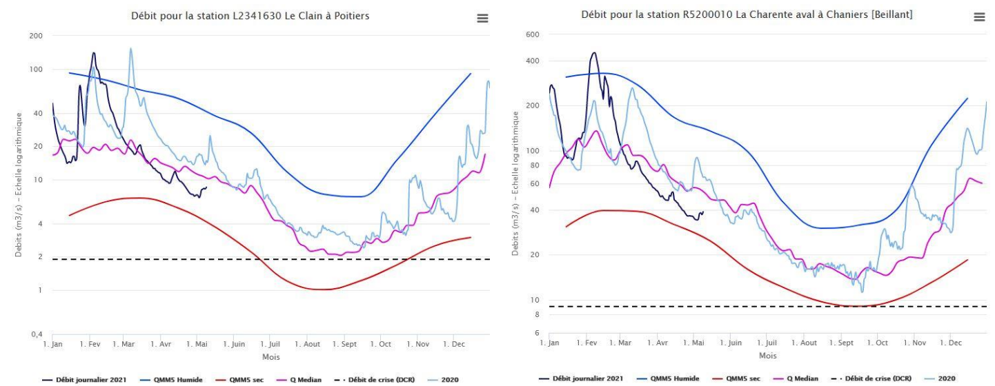
Evolution du débit de deux stations hydrométriques en 2020 et en 2021 Le Clain à Poitiers (à gauche) et la Charente aval à Chaniers (à droite)
